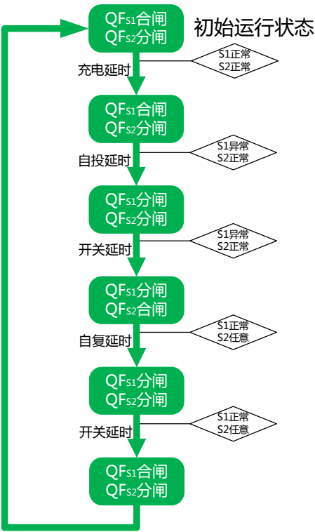
图一 2A 型控制器自投自复流程
